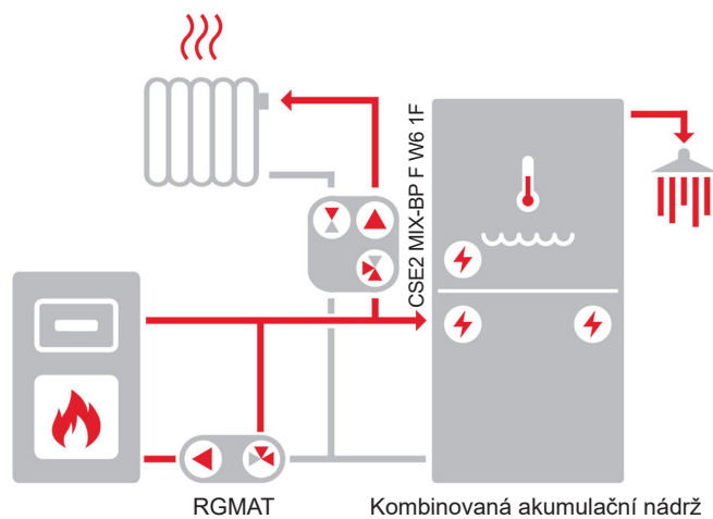
Příklad zapojení
